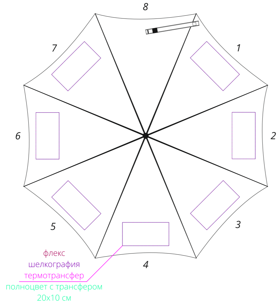
купол M1:10
